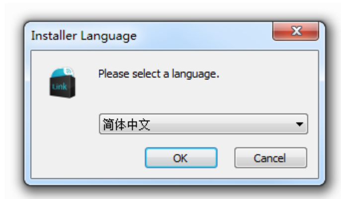
图2-2-1 安装向导
