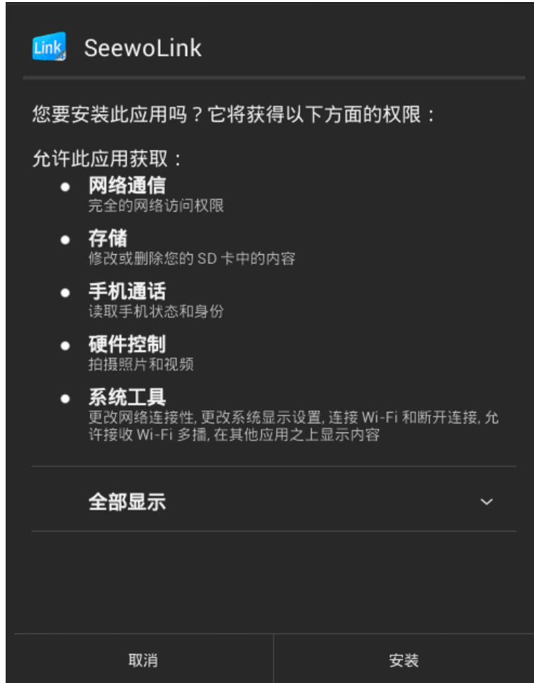
图 2-3-1 安装软件
