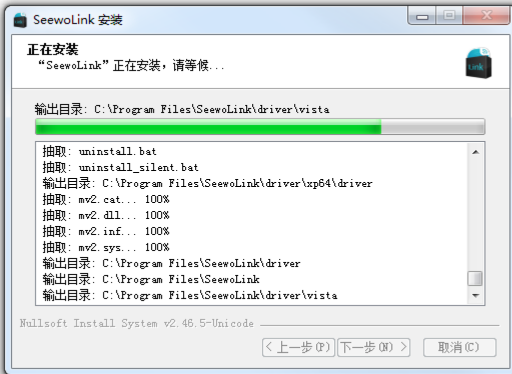
图2-2-5 安装界面
