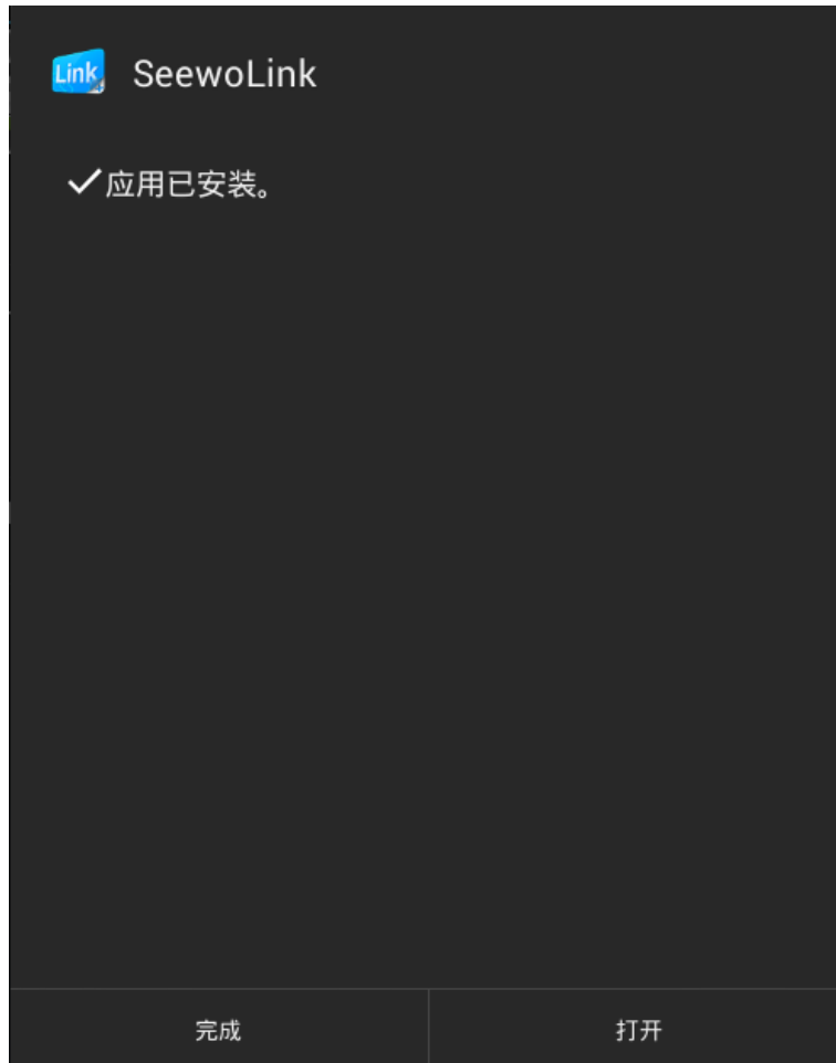
图2-3-3 安装完成
