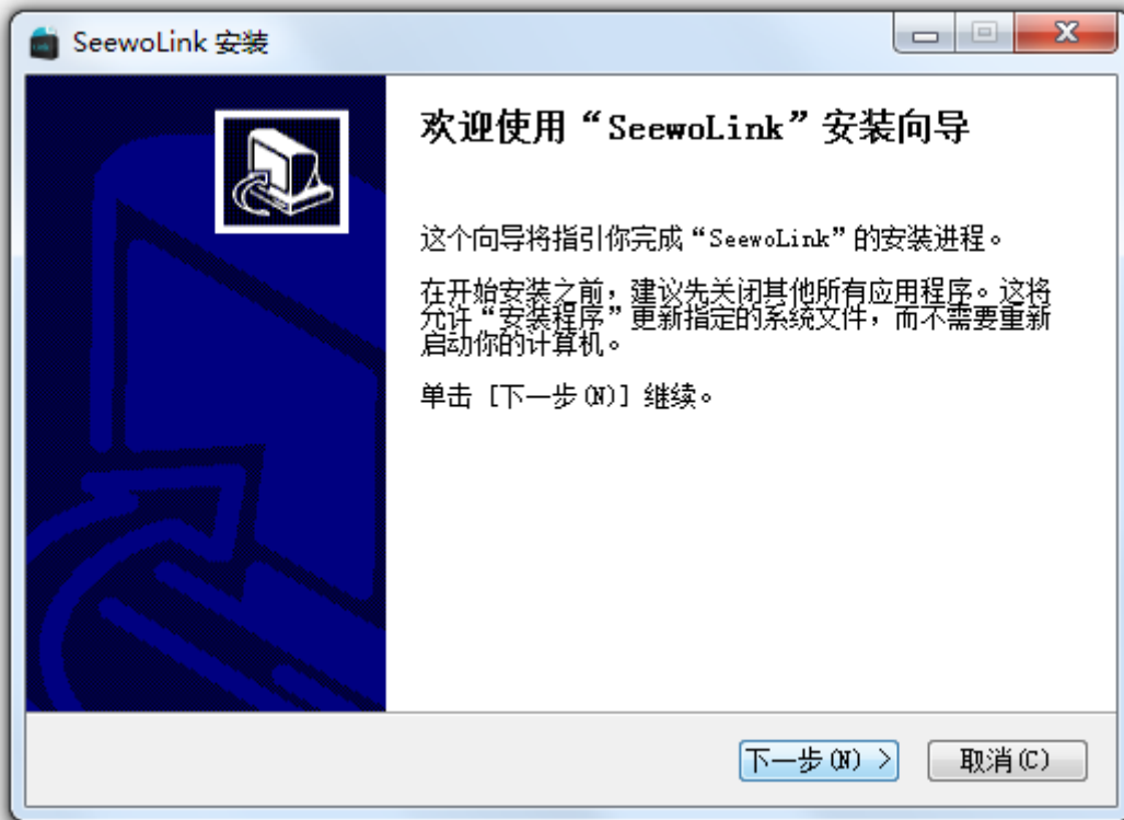
图2-2-2 安装向导
