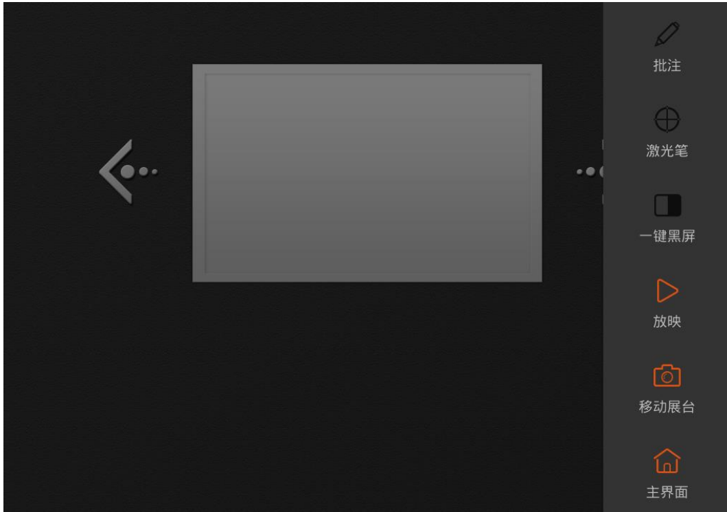
图 3-2-4-1-4 结束放映
