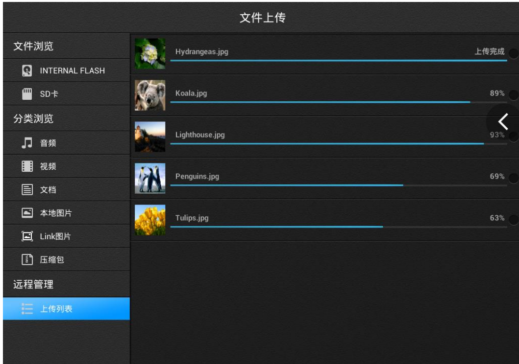
图 3-2-6-1-4 上传列表
